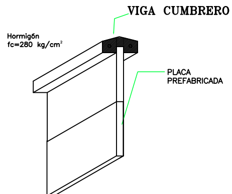
Viga Superior "Cumbrero"
