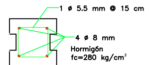
ARMADO DE COLUMNA
