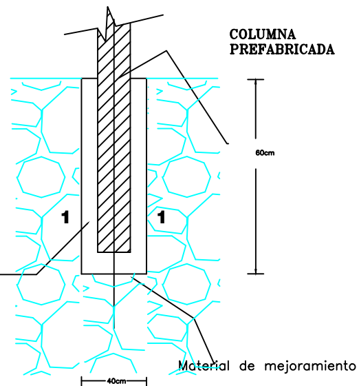
ARMADO DE COLUMNA
